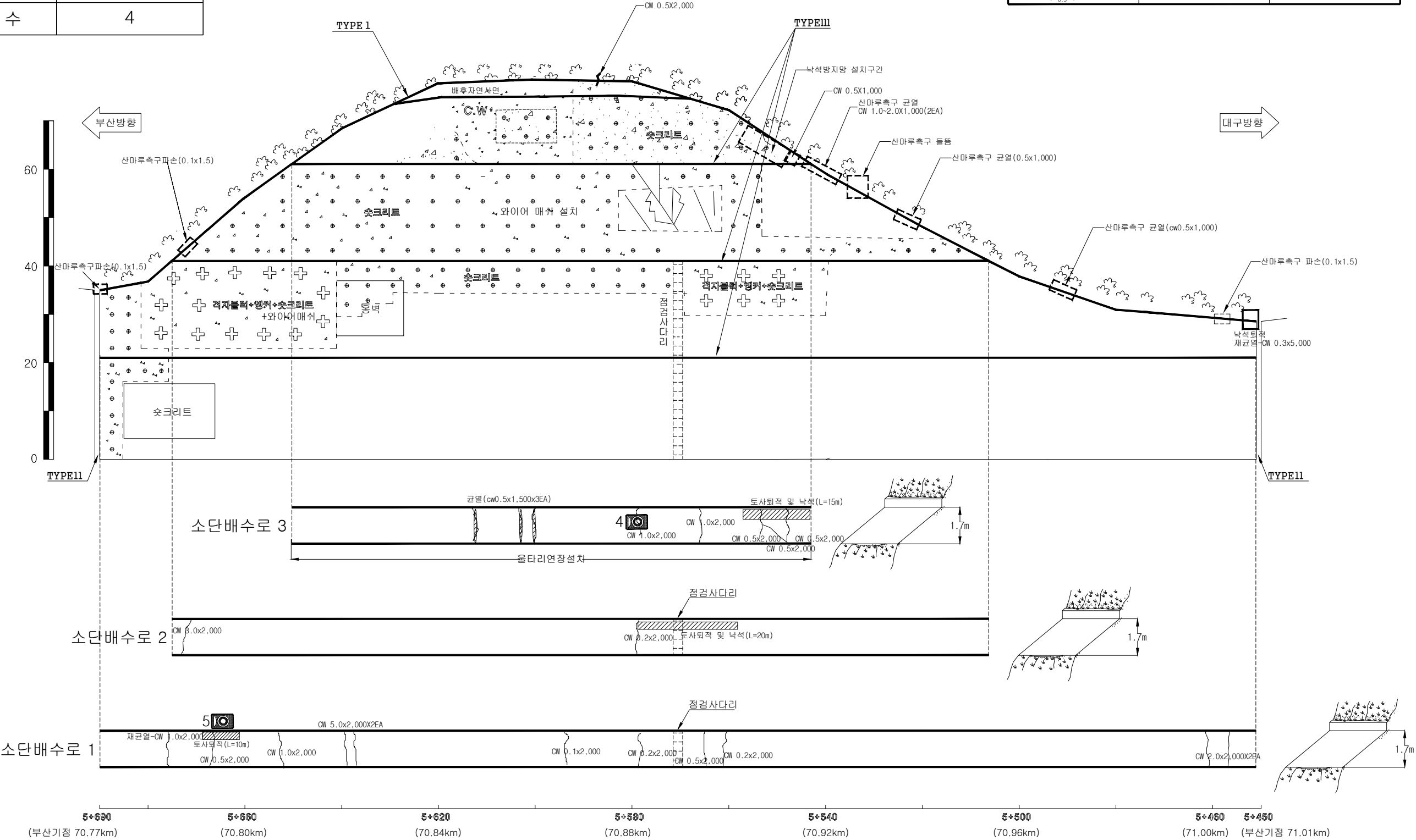
부산절토 15 / 부산기점 70.77~71.01km (4공구 STA.5+450~5+690)
